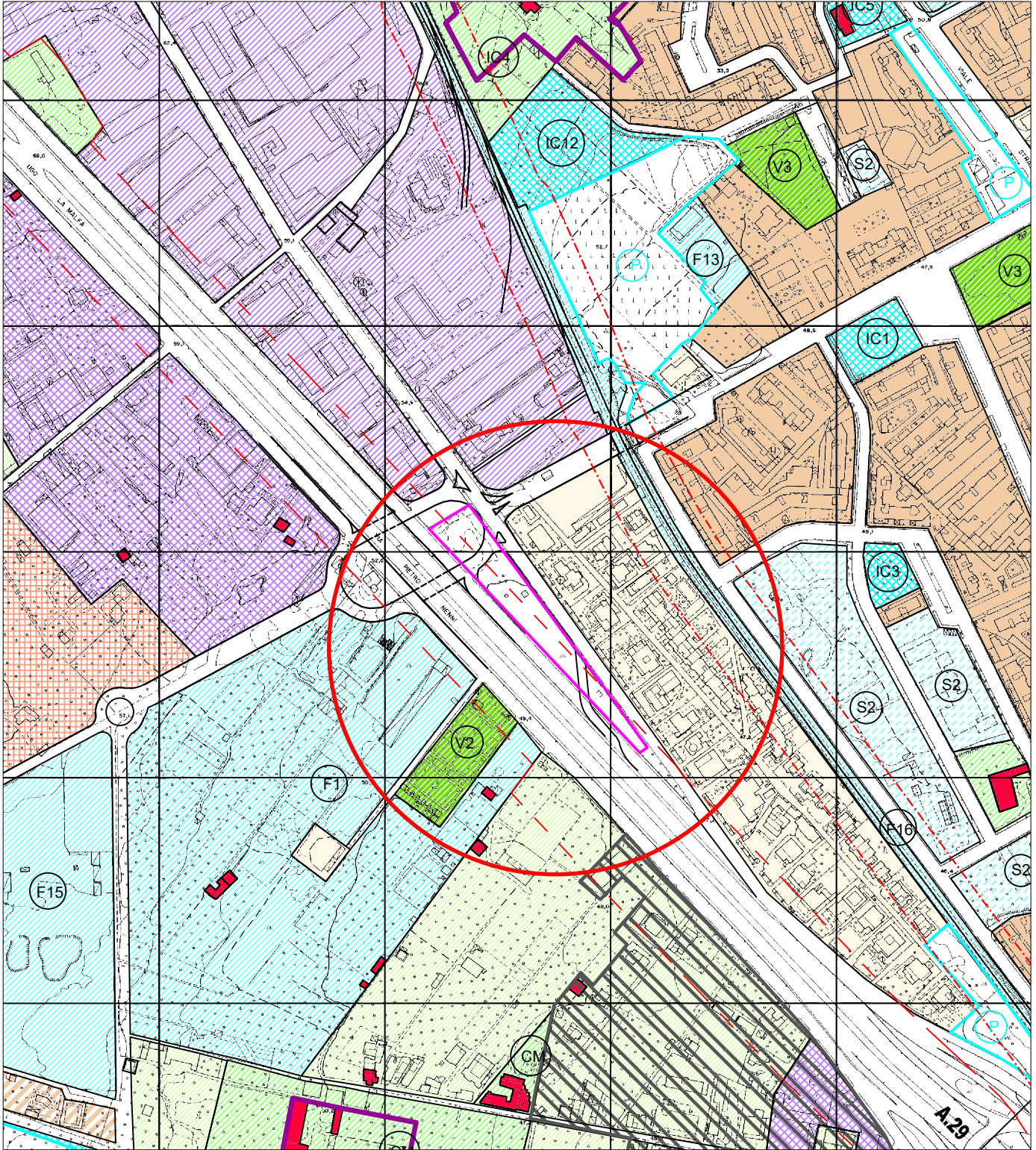
Stralcio PRG di cui alla delibera di C.C. n° 07 del 2004 Tavola P2a n° 5007 - Foglio 29 particelle 3259, 3261 3262, 3263 e 3264 - STATO ATTUALE - scala 1:5000
