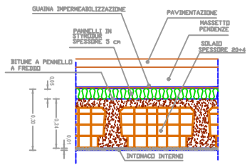
PARTICOLARE SOLAIO DI COPERTURA
