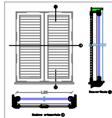
PARTICOLARE INFISSO ESTERNO
