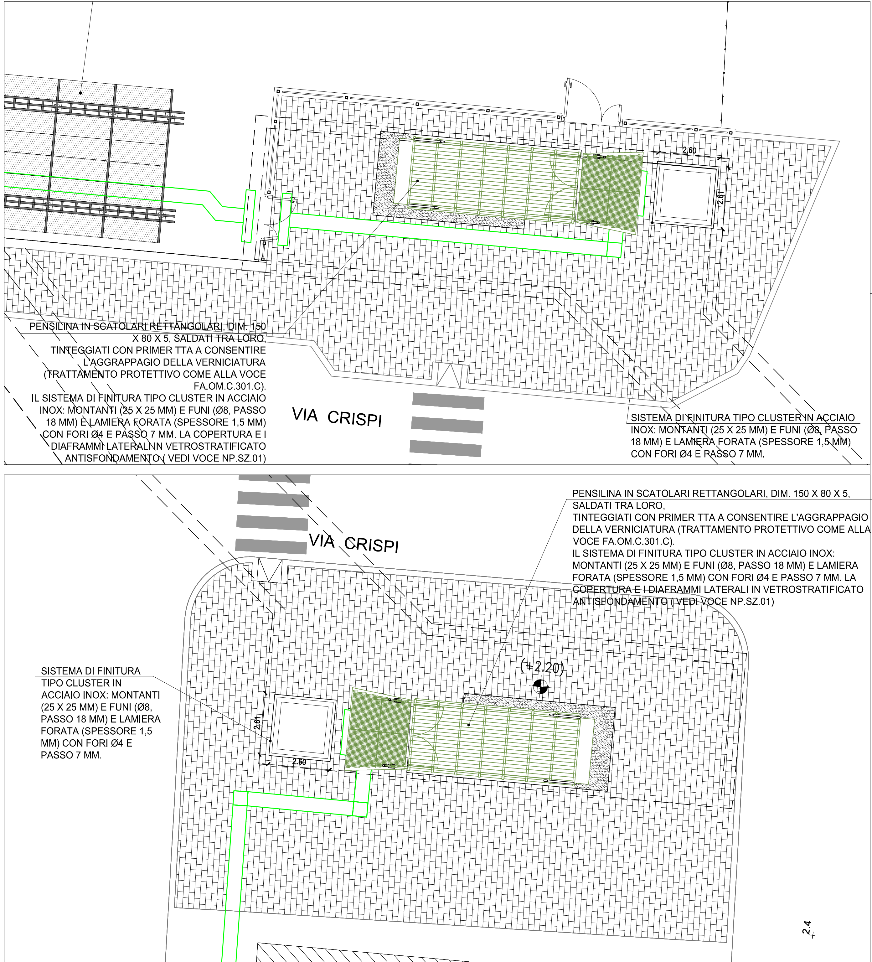
PIANTE COPERTURA [sottopasso] scala 1:100
