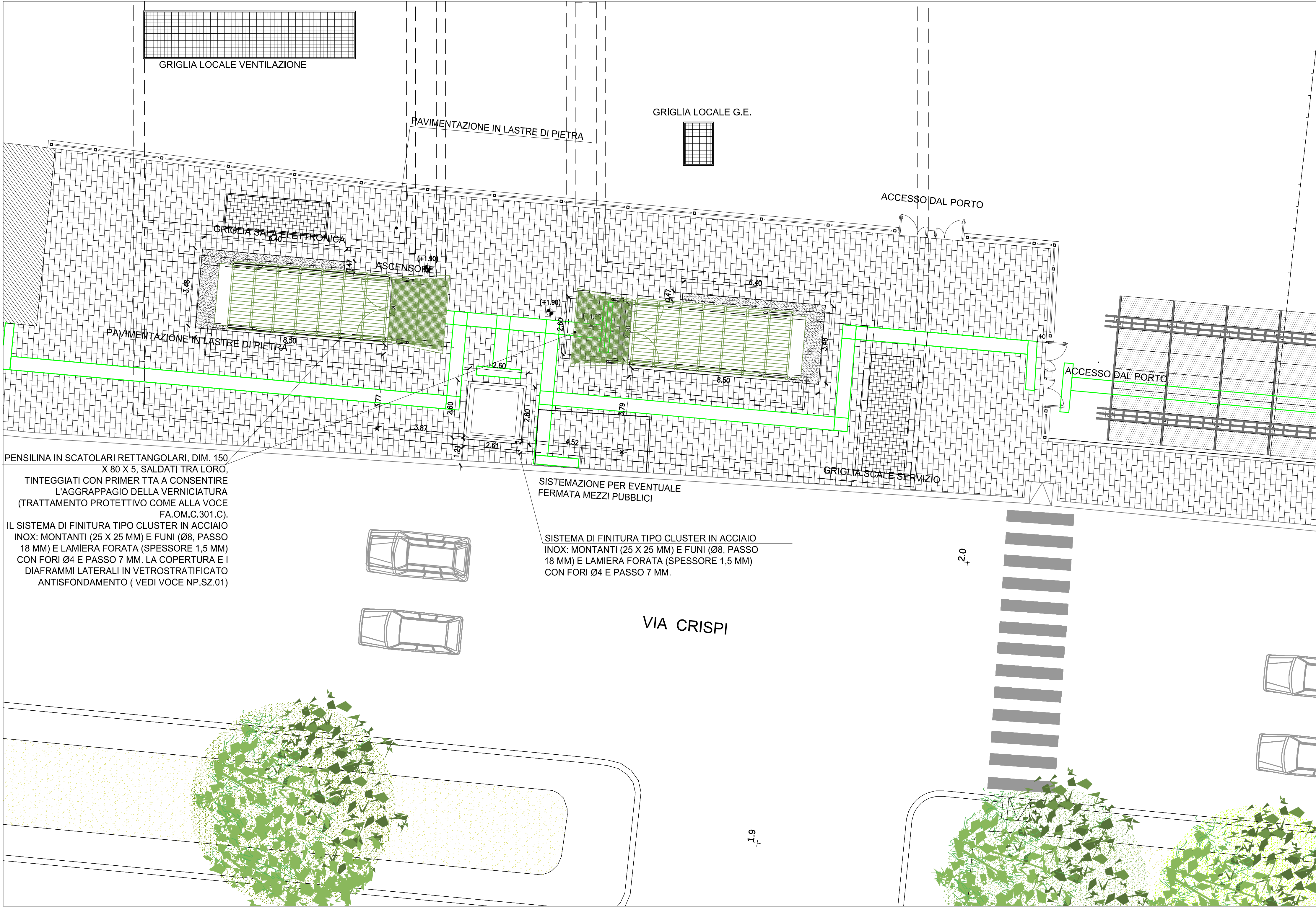
PIANTA COPERTURA LIVELLO ACCESSI scala 1:100
